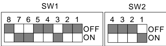
23. AMD-K6/233 (3.2V)
