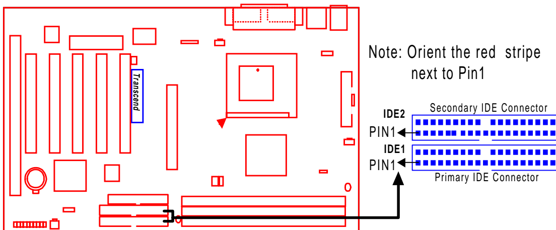
IDE Connectors
