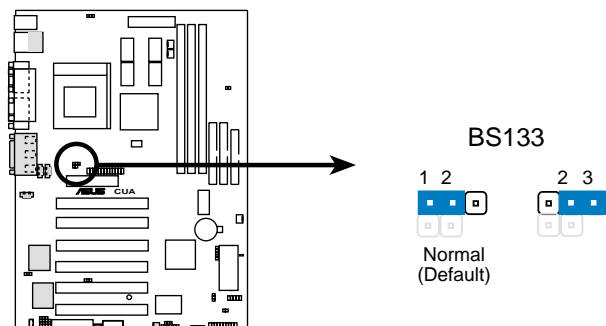
CUA Bus Selection
