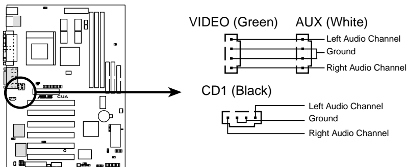
CUA Internal Audio Connectors
