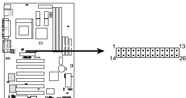
CUA Feature (VMI) Connector
