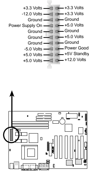
CUA ATX Power Connector
