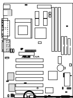
CUA Wake-On-LAN Connector
