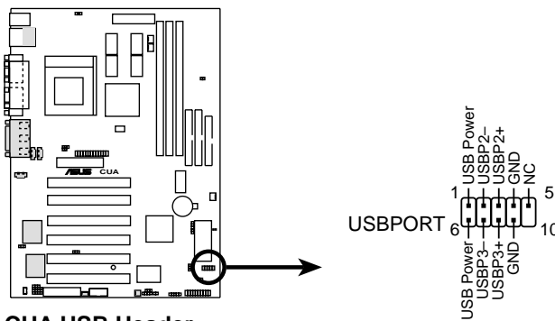
CUA USB Header
