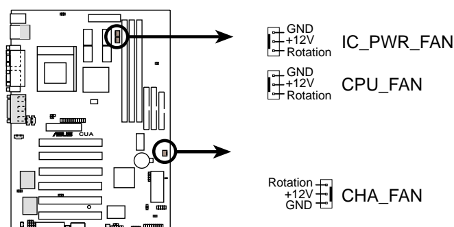
CUA 12-Volt Cooling Fan Power
