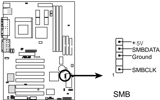
CUA SMBus Connector
