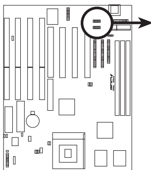
Anschluß für serielle Schnittstellen
