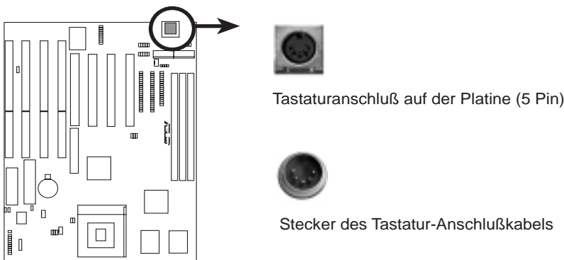
Tastaturanschluß
