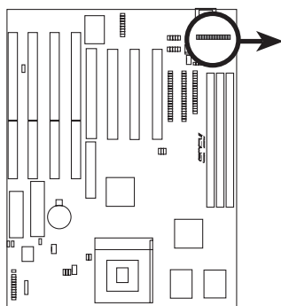
Anschluß für die parallele Schnittstelle
